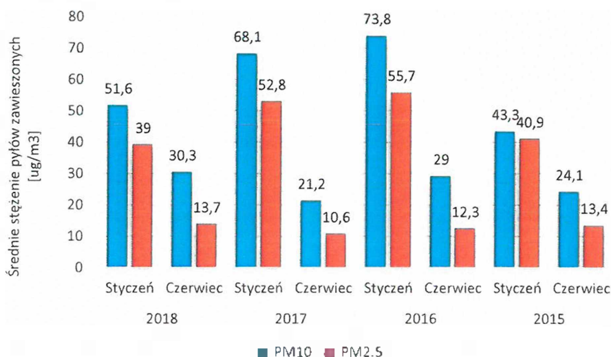
Wykres 12 Średnie stężenie pyłów zawieszonych [ \mu\text{g}/\text{m}^3 ] dla stycznia i czerwca w latach 2015-2018 odnotowane na stacji pomiarowej MzŻyraRoosev (Żyrardów-Roosevelta), na podstawie Bazy Danych GIOŚ
