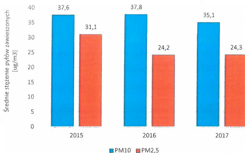
Wykres 11 Średnie stężenie pyłów zawieszonych [ \mu\text{g}/\text{m}^3 ] w latach 2015-2017 odnotowane na stacji pomiarowej MzŻyraRoosev (Żyrardów-Roosevelta), na podstawie Bazy Danych GIOŚ.
