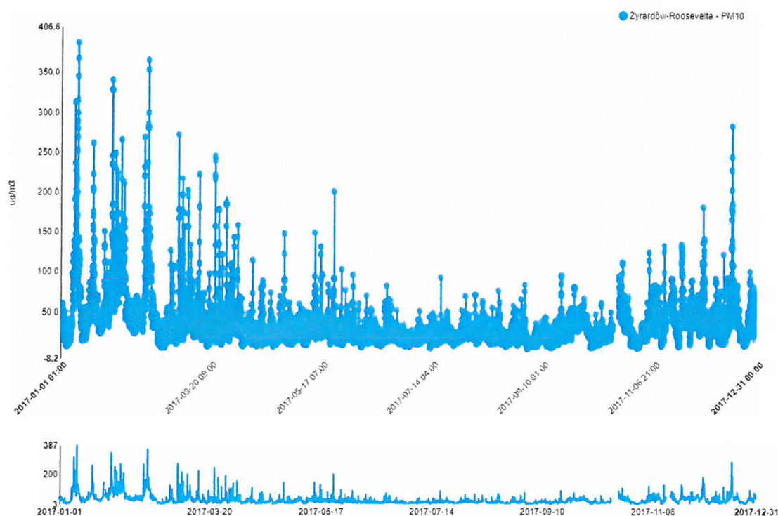
Wykres 5 Wyniki pomiarów ze stanowiska MzŻyrardów (Żyrardów Roosevelt) dla pyłu zawieszonego PM10 w okresie styczeń 2017 – grudzień 2017 w trybie automatycznym. Wygenerowane na podstawie banku danych pomiarowych Inspekcji Ochrony Środowiska.
