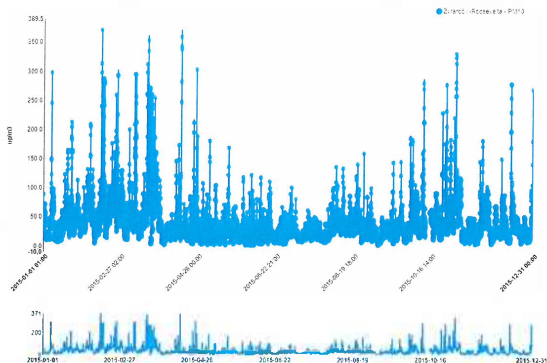
Wykres 7 Wyniki pomiarów ze stanowiska MzZyraRoosev (Zyrardów Roosevelta) dla pyłu zawieszonego PM10 w okresie styczeń 2015 – grudzień 2015 w trybie automatycznym. Wygenerowane na podstawie banku danych pomiarowych Inspekcji Ochrony Środowiska
