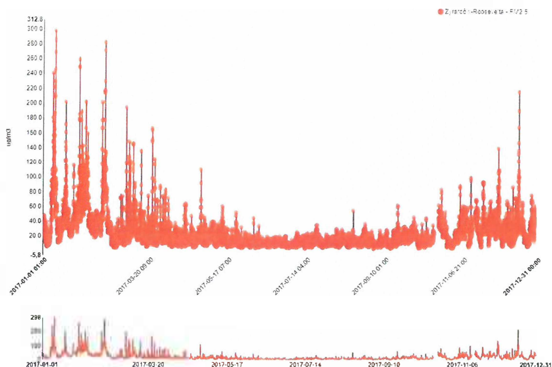
Wykres 8 Wyniki pomiarów ze stanowiska MzŻyraRoosev (Żyrardów Roosevelt), dla pyłu zawieszonego PM2.5 w okresie styczeń 2017 – grudzień 2017 w trybie automatycznym. Wygenerowane na podstawie banku danych pomiarowych Inspekcji Ochrony Środowiska
