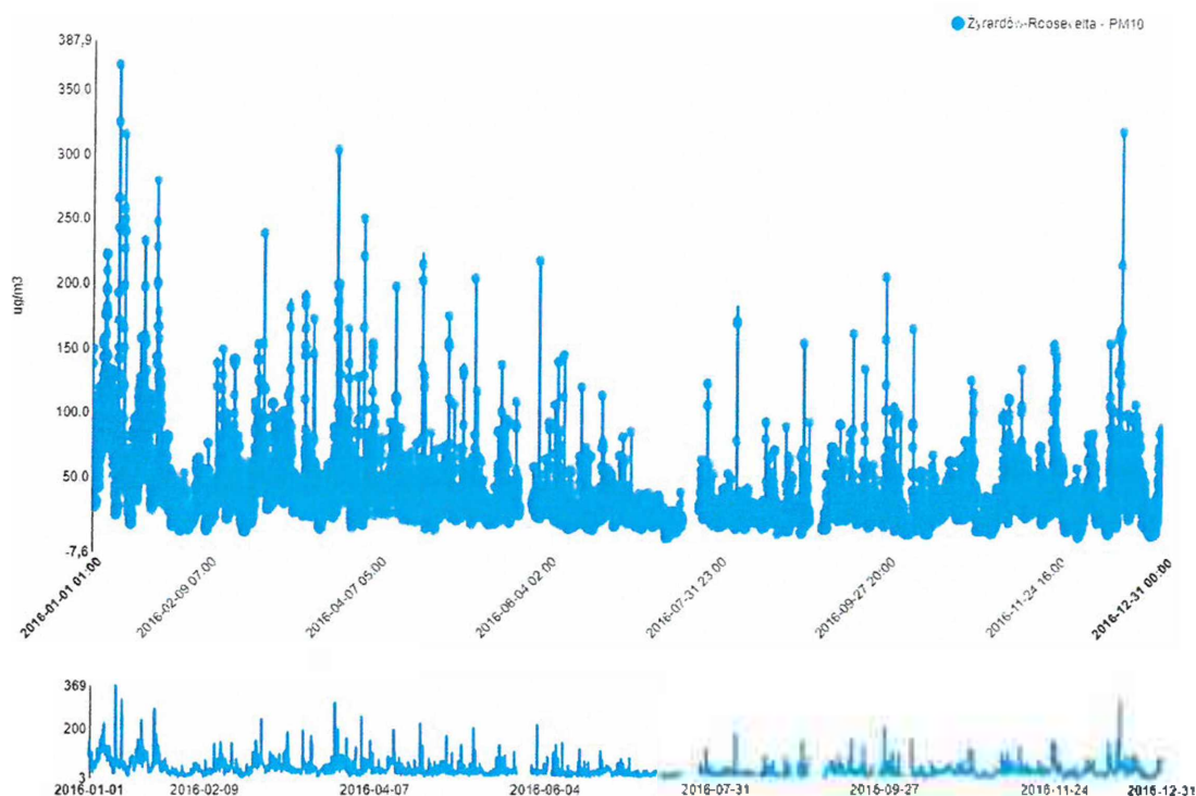
Wykres 6 Wyniki pomiarów ze stanowiska MzZyraRaosev (Zyrardów-Roosevelta) dla pyłu zawieszonego PM10 w okresie styczeń 2016 – grudzień 2016 w trybie automatycznym. Wygenerowane na podstawie banku danych pomiarowych Inspekcji Ochrony Środowiska.
