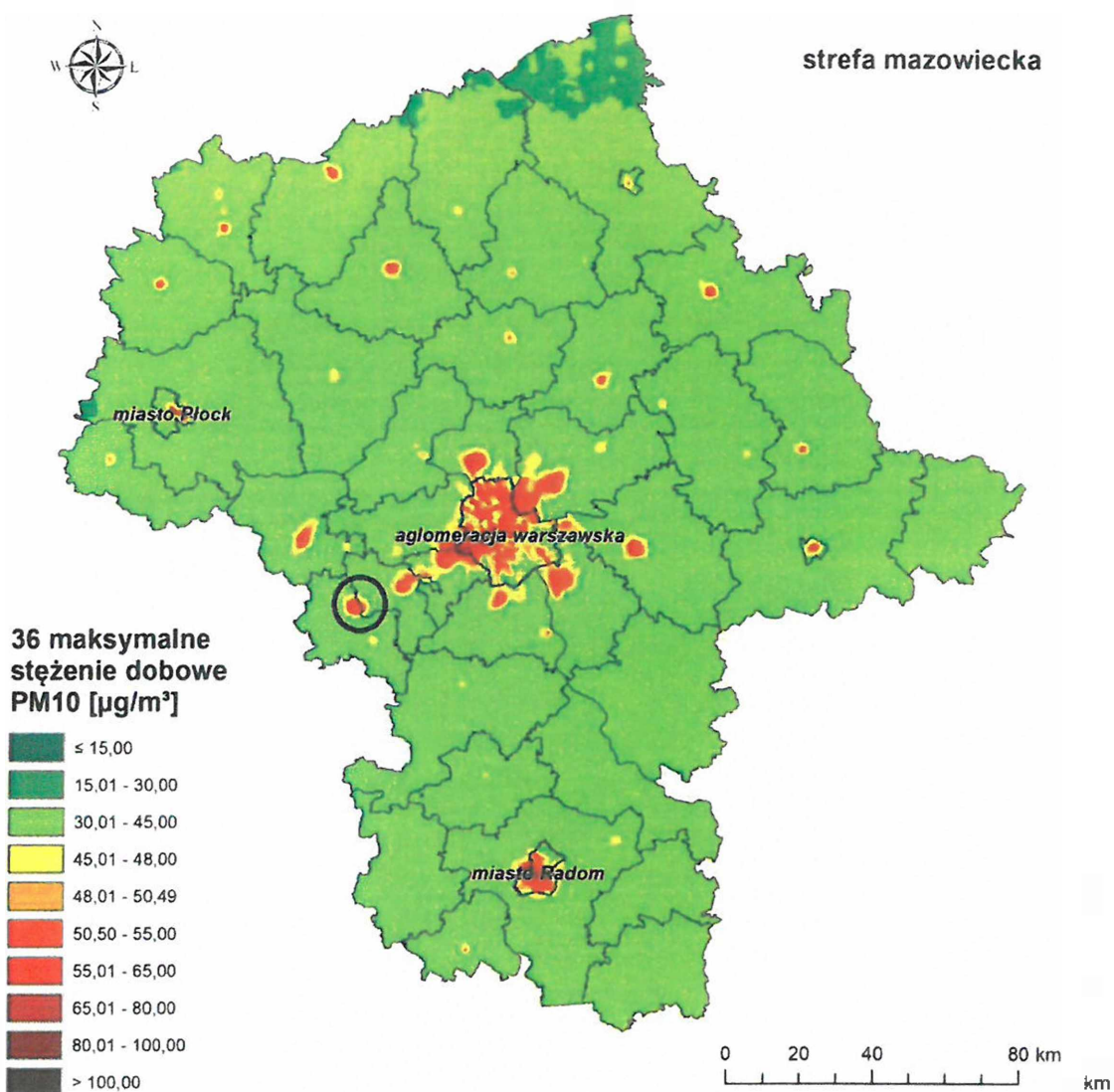
Rysunek 5 Rozkład stężeń PM10-24h (36 te maksimum w roku) na obszarze województwa mazowieckiego, cel: ochrona zdrowia (rok 2017) Za: raport za rok 2017
