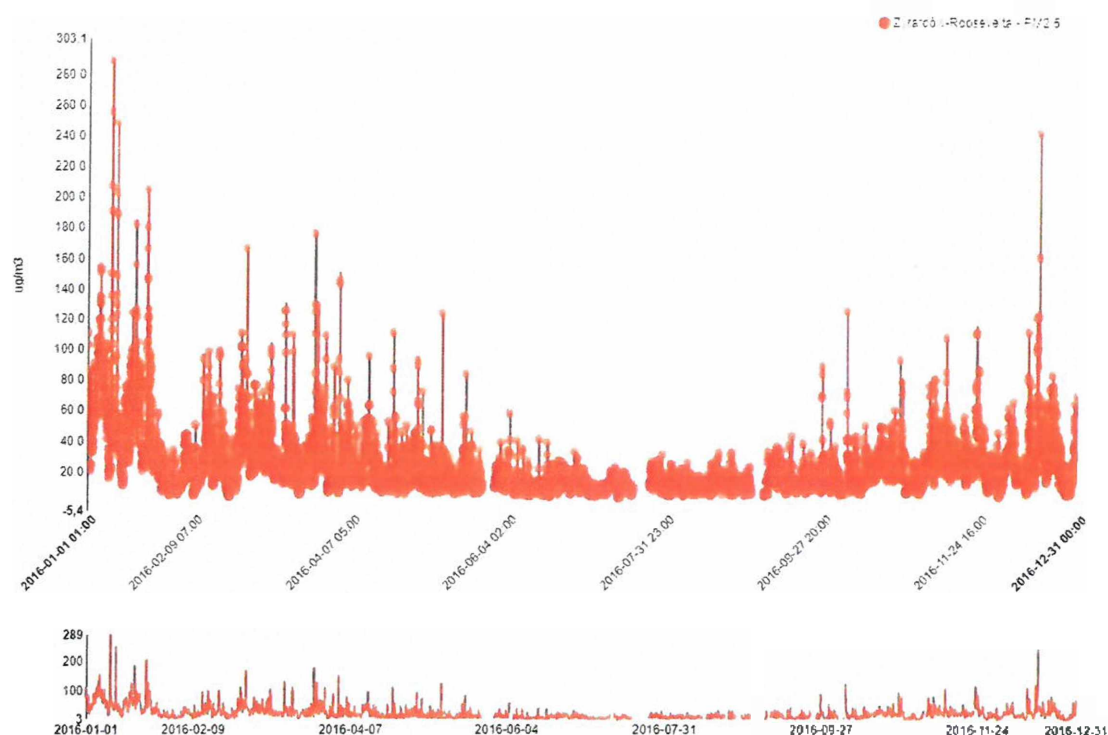
Wykres 9 Wyniki pomiarów ze stanowiska MzŻyraRoos (Żyrardów Roosevelt) dla pyłu zawieszonego PM 2.5 w okresie styczeń 2016 – grudzień 2016 w trybie automatycznym. Wygenerowane na podstawie banku danych pomiarowych Inspekcji Ochrony Środowiska.
