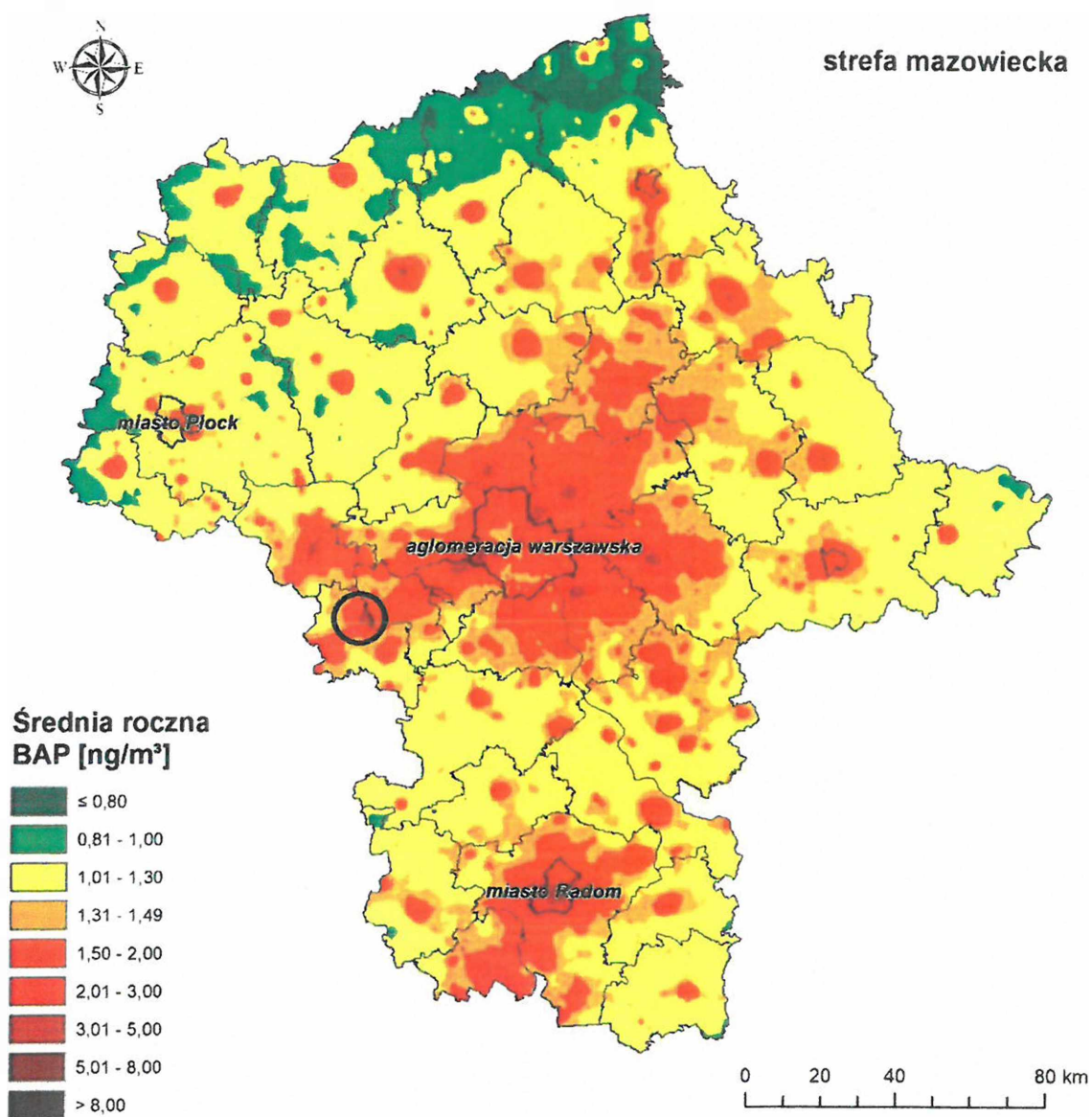
Rysunek 3 Rozkład stężeń benzo(a)pirenu – stężenia roczne w 2017 r. ze Roczna Ocena Jakości Powietrza w województwie mazowieckim. Raport za rok 2017.
